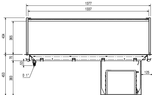
Zij aanzicht
